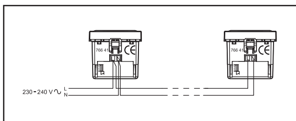
CAT XLP917WEWE wiring
