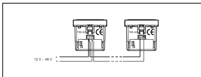
CAT XLP918WEWE wiring
